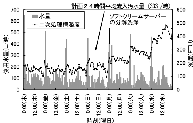
図-1 使用水量と濁度の経時変化 (A-2)
