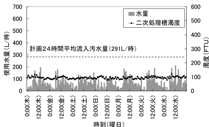
図-2 使用水量と濁度の経時変化 (B-3)
